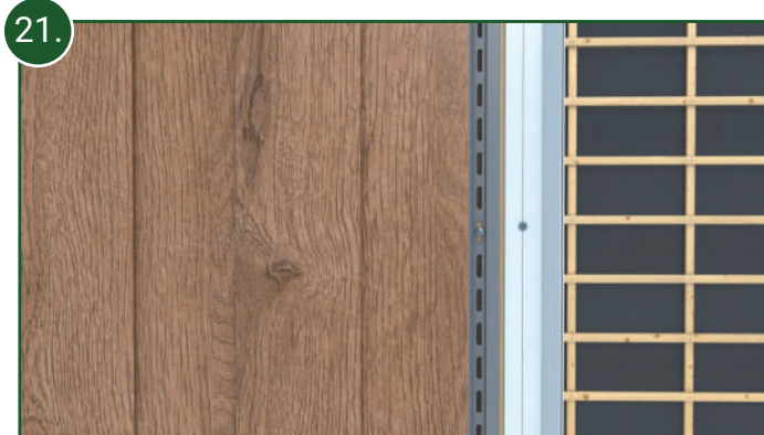
21. Das letzte Brett am Rand der Fassadenfläche muss in den meisten Fällen längsseitig gekürzt werden.
