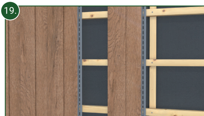
19. Die Fassadenprofile werden nach dem vorgenannten Schema nun schrittweise längsseitig nebeneinander montiert.
